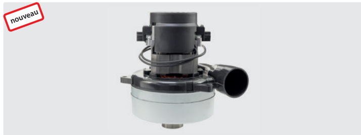
À 2 étages avec tuyère latérale et tuyère verticale. 24 V. Avec câbles préinstallés
