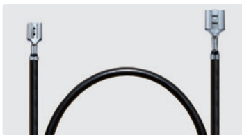
Flachhülse 6,3 : Flachhülse 4,8. Kabel 500 mm. Typ 1
