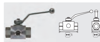
AISI 316 Ti. Poignée zinguée. Sphère en inox. Type L. Max. 100 °C
