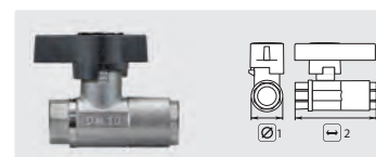
Laiton cadmié. Sphère chromée. Max. 210 bar / 80 °C
