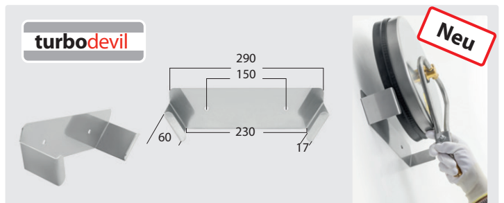
Wandhalterung Wandreiniger turbo- devil.
