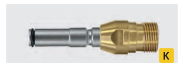
ST-247 : TR22 M. Laiton/inox. Max. 400 bar / 150° C
