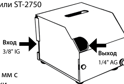
Возможные исполнения: встроенные пистолеты ST-2605 с 350 bar или ST-2750 с 500 bar
