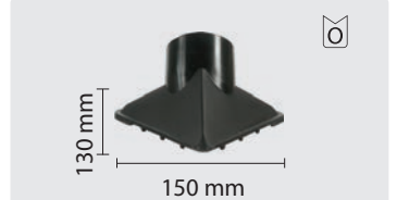
Dreiecksdüse
