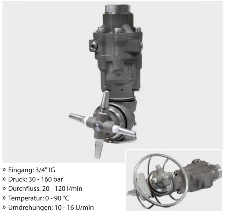
ST-82 h16/120 Selbstdrehender Tankreiniger
