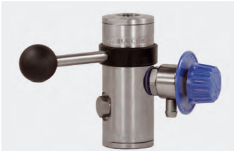
Injecteur by-pass ST-167 avec doseur ST-161, cannelé 9 mm
