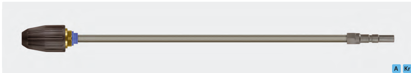
Coupleur KW. Lances tube zingué avec rotabuse ST-456. Cône 20°. 200 - 350 bar. Max. 100 °C
