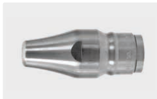
1/4" IG. 300-600 bar. Max. 90 °C
