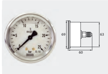
∅ 63 mm. Boîtier inox. 1/4" M. Entrée latérale: Type WIKA
