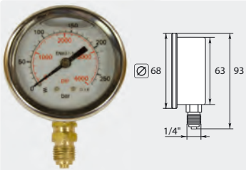
∅ 68 mm. Boîtier inox. 1/4" M. Entrée verticale
