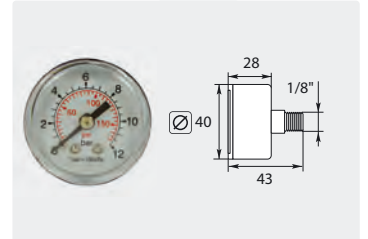
∅ 40 mm. Boîtier PVC. 1/8" M. Entrée latérale
