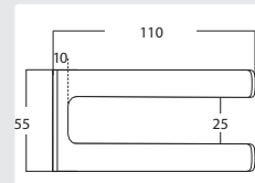
Edelstahlhalter für Wandmontage
