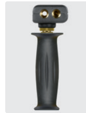
Ventil seitlich. Max. 310 bar / 150 °C
