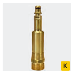
Coupleur mâle 8,8 : M22 M. Laiton. Max. 250 bar / 100 °C
