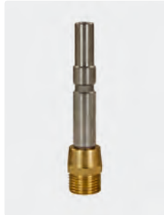
Coupleur mâle KW inox : M22 M. Laiton. Pour lances avec raccord manuel
