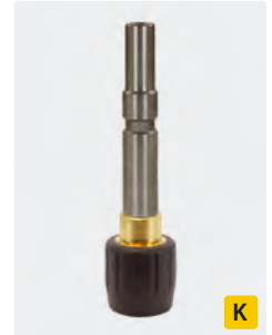
Coupleur mâle KW inox : porte-buse pastille sans buse. Max. 400 bar / 150 °C
