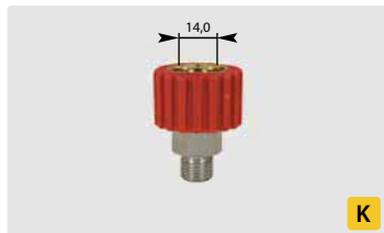
M22 F : M. Max. 250 bar / 120 °C
