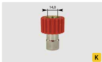
M22 F : F. Max. 250 bar / 120 °C
