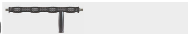
1/4" AG. Strahlrohr mit Griff und Isolierung ST-28.2/ST-29.2 Cool & Compact. Max. 400 bar / 150 °C
